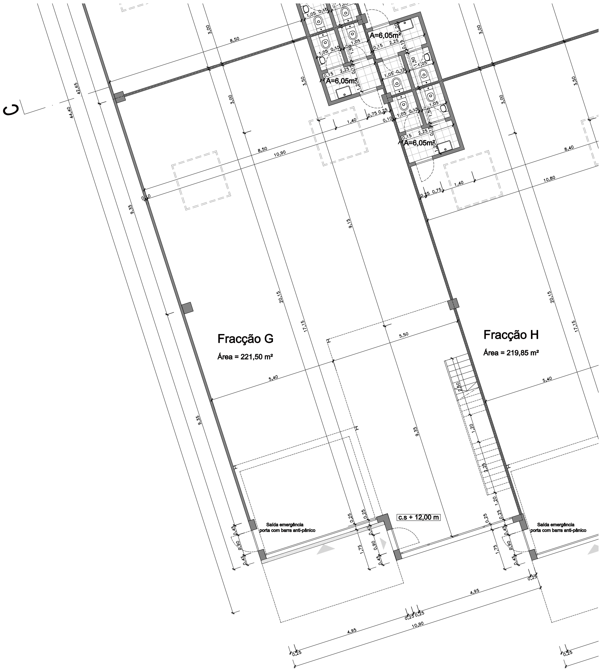
PLANTA PISO 0
