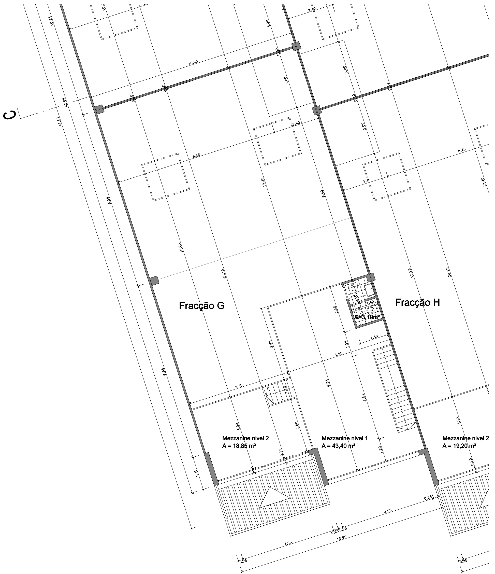
PLANTA PISO 1
